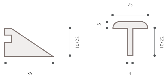
RACCORDO E GIUNTO DI DILATAZIONE
